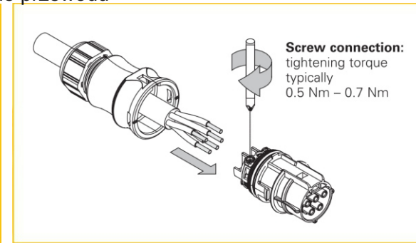
Podłączenie przewodu
