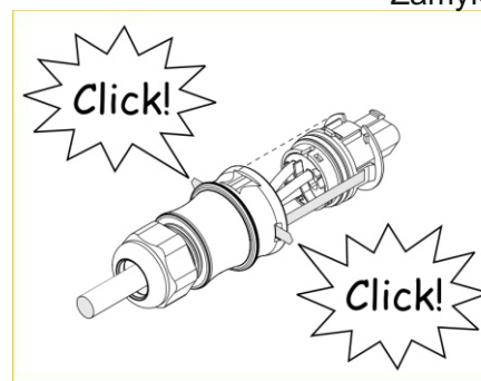
Zamykanie RST
