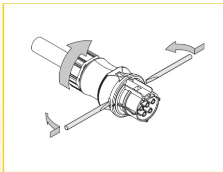
Otwieranie RST
