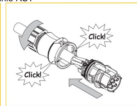
Zamykanie RST
