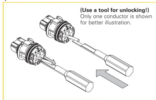
Odłączenie przewodu
