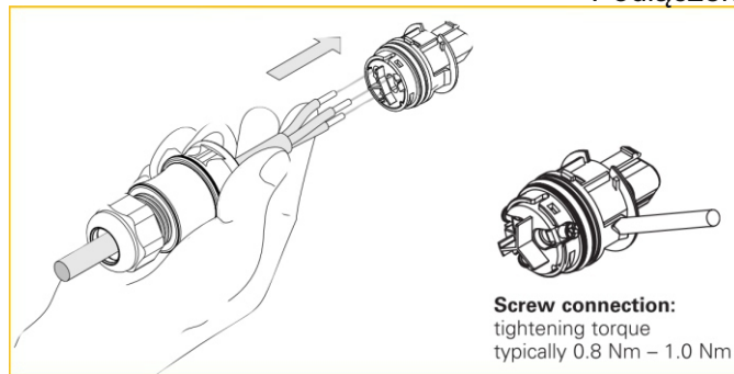
Podłączenie przewodu
